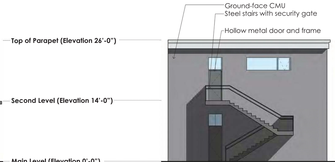
North Elevation Scale: 1/8" = 1'-0"
